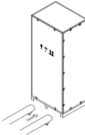
Рисунок 2.1 Перемещение оборудования
