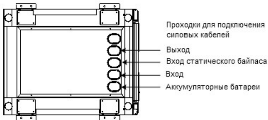
Рисунок 2.5. Проходки для ввода кабелей ИБП 10 кВА – 60 кВА
