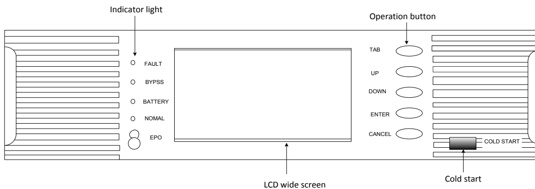
Рисунок 3.1 Панель управления
