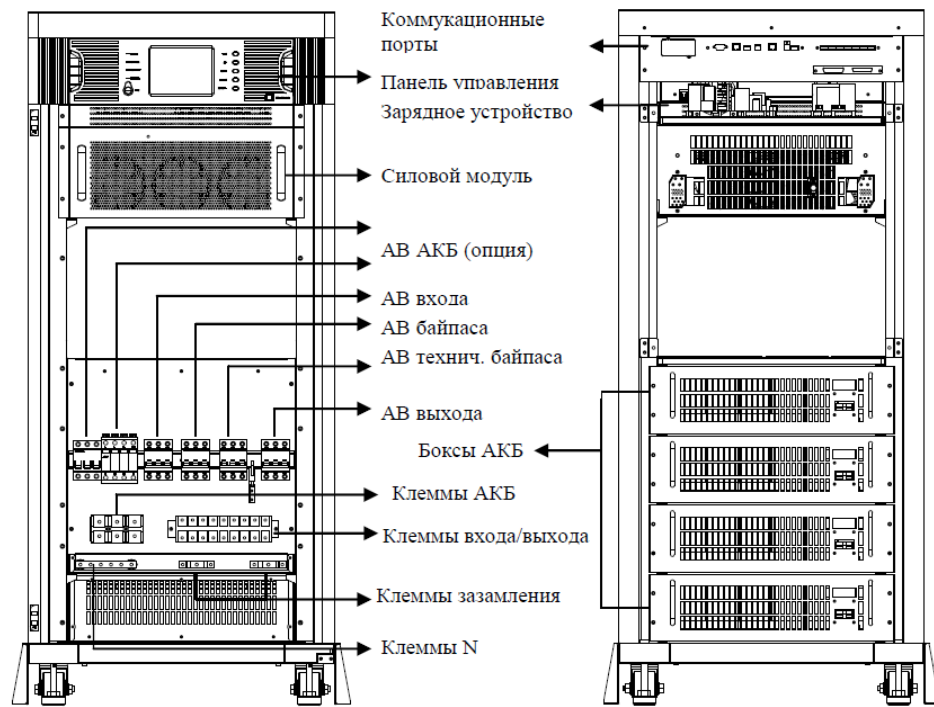
Фронтальный вид (без двери и защитных панелей)
