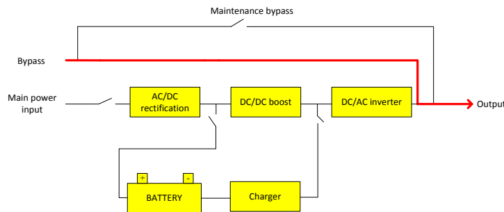
Рисунок 1.5 Схема работы в режиме байпаса
