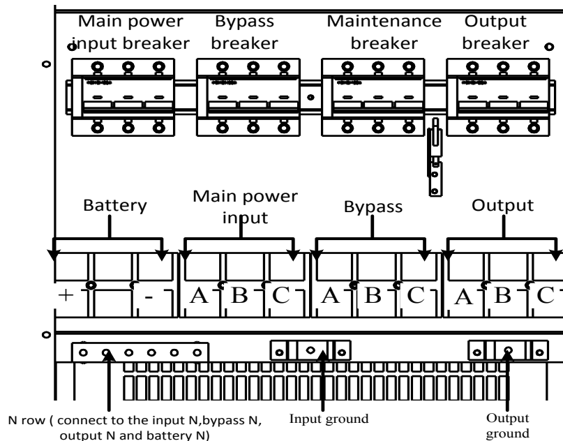
Рисунок 2.11. Расположение контактных выводов ИБП 40 кВА и 60кВА
