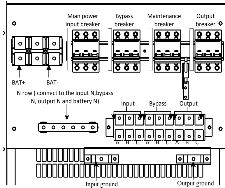
Рисунок 2.10. Расположение контактных выводов ИБП 10 кВА - 30кВА
