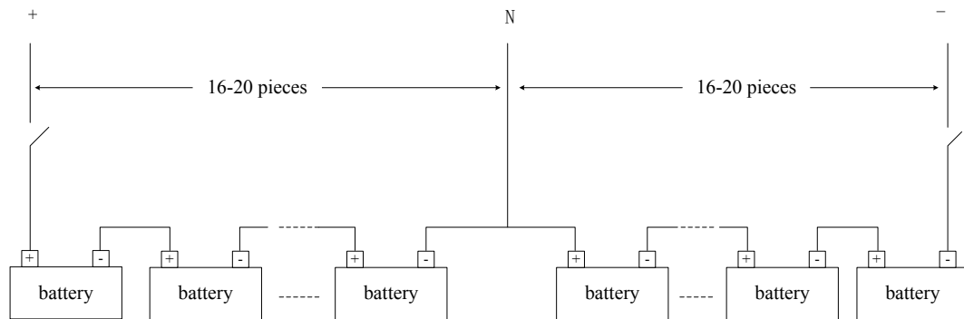
Рисунок 2.13. Схема подключения батарей
