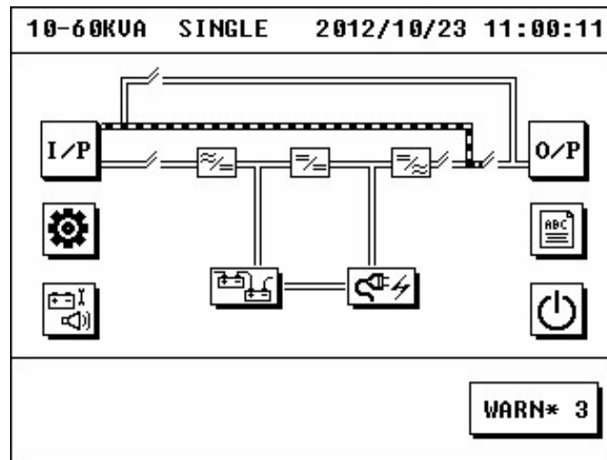
Рисунок 3.3 Основной интерфейс
