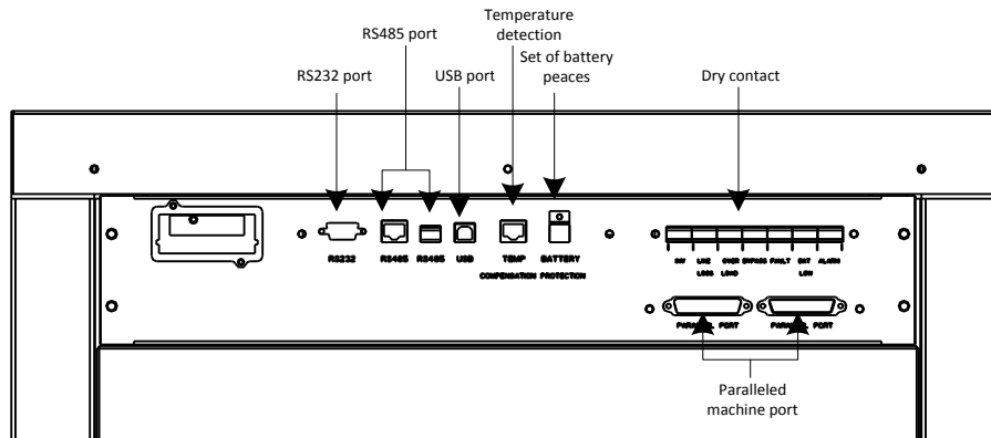
Рисунок 1 Коммуникационные порты L900II 3/3 10 кВА – 120 кВА
