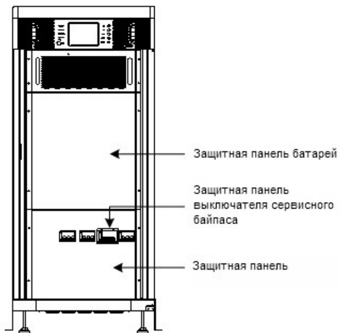
Рисунок 2.7. Вид спереди (дверь ИБП открыта) 10 кВА – 30 кВА
