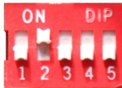
Рисунок 2 Переключатели установки адреса силовых модулей
