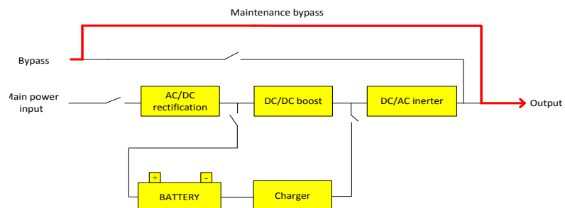
Рисунок 1.6 Схема работы в режиме технического обслуживания
