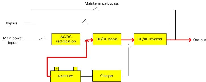
Рисунок 1.4 Схема режима работы от батарей
